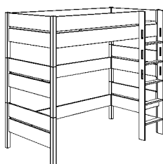
Hochbett mit Griffeiter, gerade
