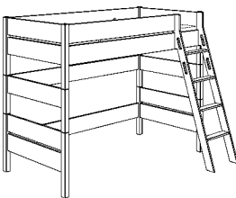
Spielbett mit Grifflleiter, schräg
